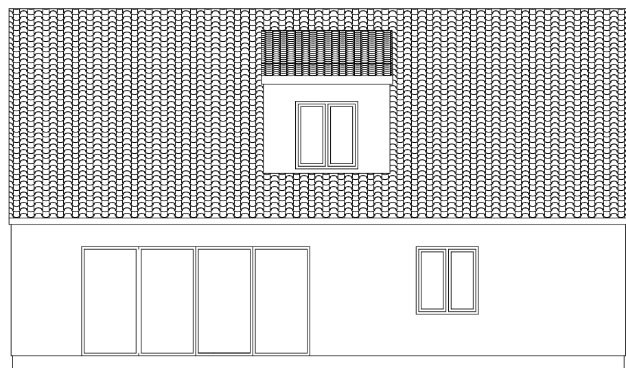
Fasad A3 1:100
